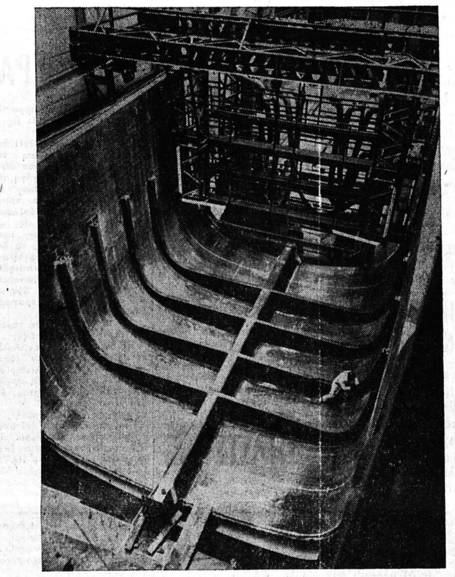
Σκάφη πλοίων των 1.000 τόννων από ίνας ύαλου. Αυτή είναι ή πλεον πρόσφατος τεχνική πρόσδος εις τήν Βρεττανίαν. Εις τήν φωτογραφία δοκιμαστικόν τμήμα σκάφους ενός πλοίου των 600 τόννων.
