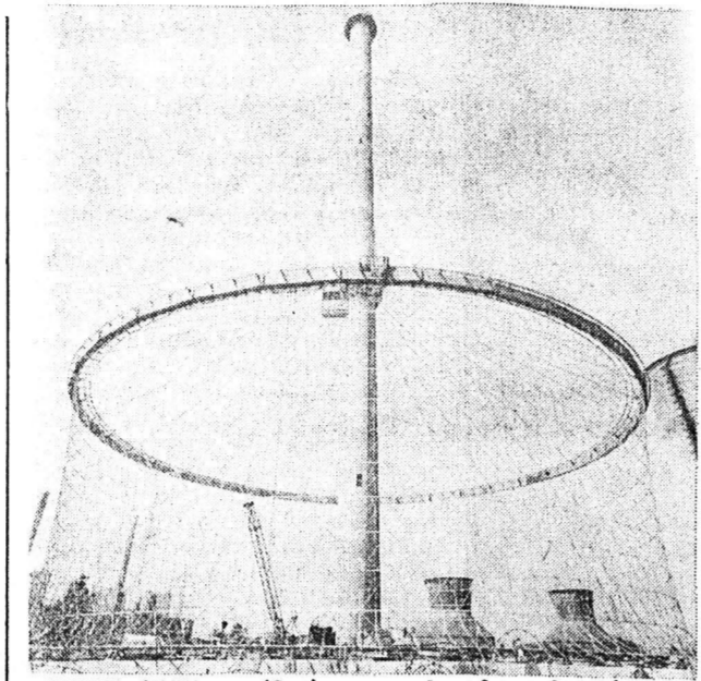
ΕΞΕΣΗ (INB) — Ο εικονιζόμενος φωτικός πύργος κατεσκευάσθη από τήν εταιρεία Φρήντριχ Κρούπ του Έσσεν για τού Ισχύος 300 Μεγαβάτ ά τομικών έργοστάσιον παραγωγής ηλεκτρικής ένεργείας τής περιοχής Ουντροπ Σμετχάου της Δυτ. Γερμανίας. Ο πύργος ύψους 180 μέτρων κρέμεται από έναν πυλώνα εκ μπετόν—άρμ, τού πλέγμα δε τού χαλιδίνου δικτύου του καλύπτεται από φύλλα άλουμινίου δε άπο τέλειαν τού βάρος όλης τής κατασκευής να μιν υπερέβαινε τού 8.000 τόνους, ενώ άν κα τεσκευάστω εκ Σιδηροκιά μάρμα θα υπερέβαινε τού βάρος τών 24.000 τόνων. Διά τού τού όμους κοστίζει και 25 εκατομμύρια μάρκα περισσότερα παρ' όσα ένας πύργος από μπετόν και τούτο διότι είναι έφασμαμένος με υδραυλικόν σύστη
