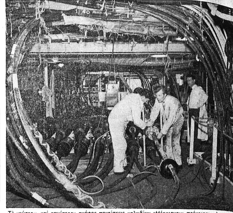
Τὸ νεότερον καὶ ταχύτερον σκάφος ποτιώσεως καλωδίων «Μέρκιουρ» πρόκειται νὰ ποτιώσῃ τὸ πρῶτον τμήμα τοῦ Κοινοπολιτευτικοῦ τηλεφωνικοῦ καλωδίου Νοτιοανατολικῆς Ἀσίας. Εἰς τὴν φωτογραφίαν ὁ θάλαμος ἐλέγχου τοῦ Μέρκιουρ.
