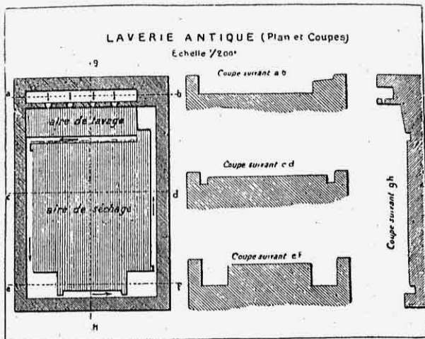
Εἰκ. 11. — Ἀρχαῖον πλυντήριον.
