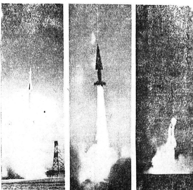
Τρεις διαφορετικοί τύποι του βλήματος «Νίκη». 'Αρι- στερά το «Νίκη-Α» εις το κέντρον το «Νίκη-Β»- ρακλήος και δεξιά το «Νίκη-Καίτηζον», το όποιον χρησιμοποιείται κυρίως εις δοκιμας άλλων βλημάτων
