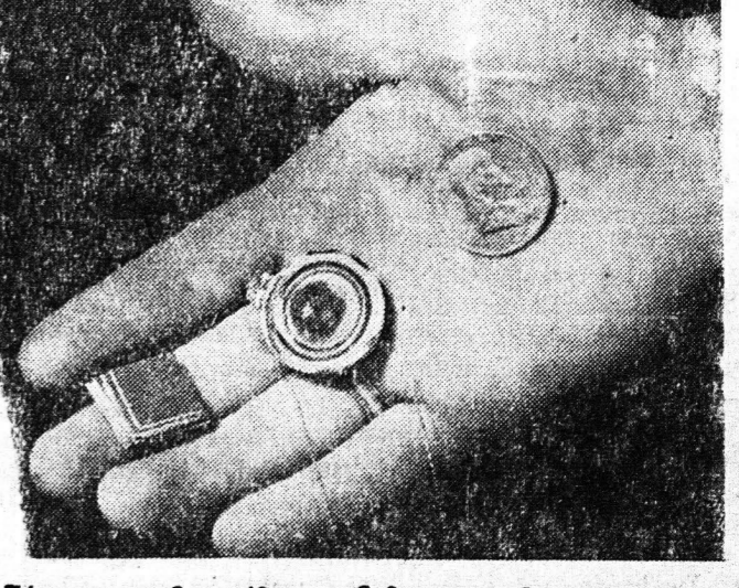
Σύγκρισις του μεγέθους του θερμιοκτικού μετατροπέως -στην μέση- με ένα νόμισμα του μισού δολαρίου. Δεξιόμα των πλοκών ραδιενεργού χρυσού, που χρησιμοποιήθη εν συνδυασμώ με τον μετατροπέα, για την παραγωγή ρευσμάτων, φαίνεται αριστερά...
