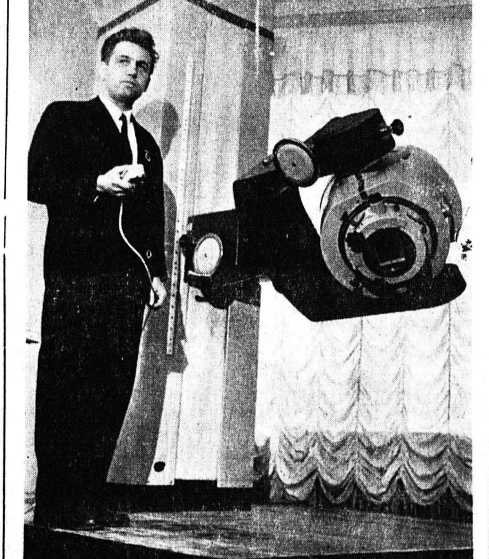
Η συσκευή «ΛΟΥΣΤ» — I» πρὸς καταπολέμησιν τοῦ καρκίνου διὰ βομβαρδισμοῦ κοβαλτίου
