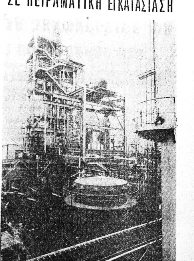
ΘΜΠΕΡΧΑΟΥΖΕΝ. Στο 'Ομπερκχάουζεν άρχισε πρόσφατα να λειτουργεί η πρώτη μεγάλη έγκατάσταση δοκιμίων για την αεριοποίηση του άνθρακος με την όποια θα δοκιμασθεί στην Δυτική Γερμανία η οικονομική παραγωγή συνθετικού φωταερίου.
