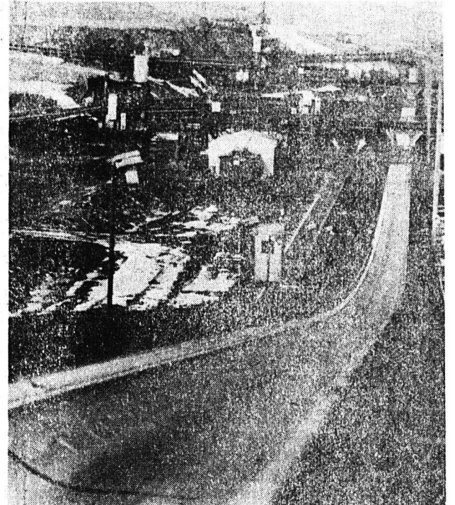
ΝΤΟΥΙ-ΣΜΠΟΥΡΚ. — Οι εγκαταστάσεις ταινίας μεταφοράς (στην φωτογραφία), που κατασκευάζονται από την ανώνυμη εταιρία Ντεμάγκ (Ντούσιμπουργκ, Δυτική Γερμανία) στην βιομηχανική περιοχή του Καναδά έχουν μήκος έντεκα χιλιόμετρα. Το σχέδιο αυτό ταινίας κατασκευαστική για μια εγκατάσταση εξαγωγής πετρελαίου από τη τρελαιφόρο άμμο που εξάγεται από μια κοινή επιχείρηση εκ-
