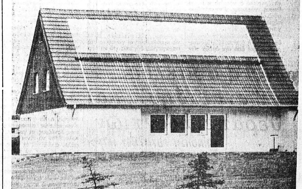
Το ήλιακό πειραματικό σπίτι στο Άαχεν, έχει έμβαδόν 120 περίπου τετραγωνικών μέτρων. Στη στέγη του έχει ειδικούς συλλέκτες για την συγκέντρωση της ηλιακής ακτινοβολίας.
